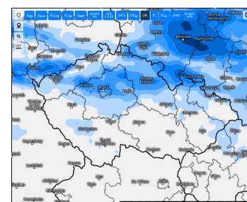
Bratr UKMO
