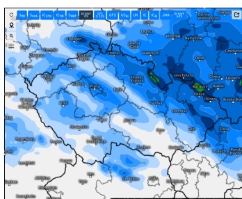
Bratr ECMWF
