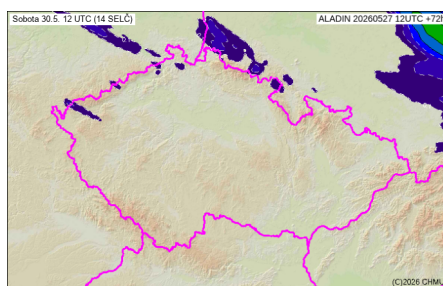
Bratr Aladin
